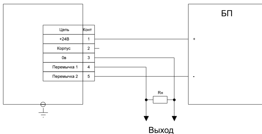
Рисунок Б.2 Схема подключения уровнемера РИЗУР-НМТ-М без взрывозащиты и и со взрывозащитой вида «взрывонепроницаемая оболочка» 4х проводная схема подключения
