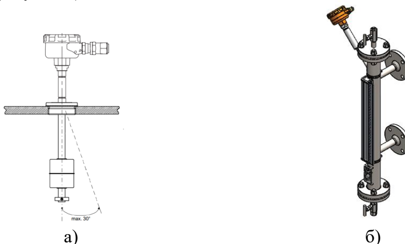
Рисунок 6 - Пример монтажа уровнемера: а) на емкости, б) на байпасной камере
