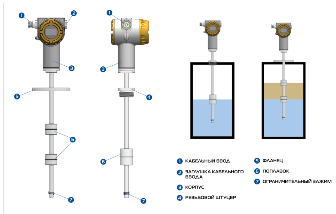
Рисунок 2 – Устройство уровнемера
