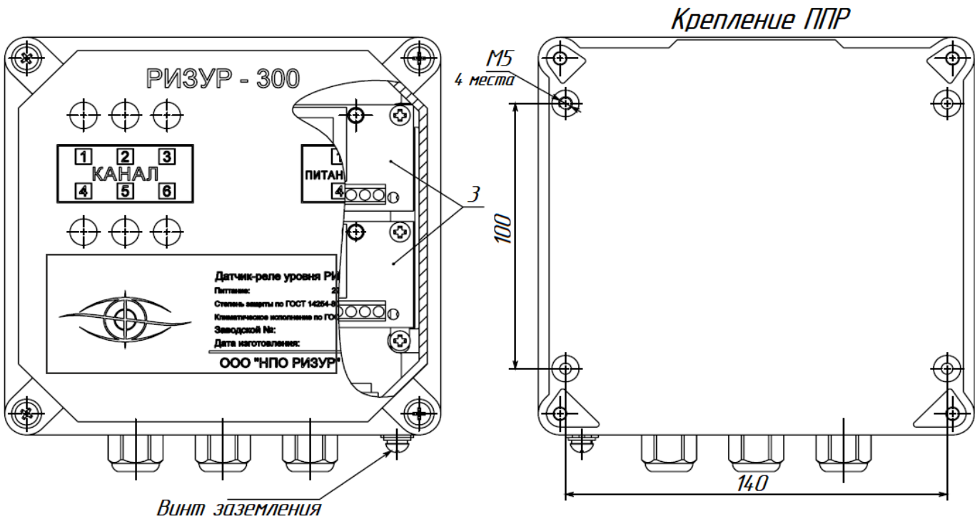
Рис.2.2. 4-6 датчика
