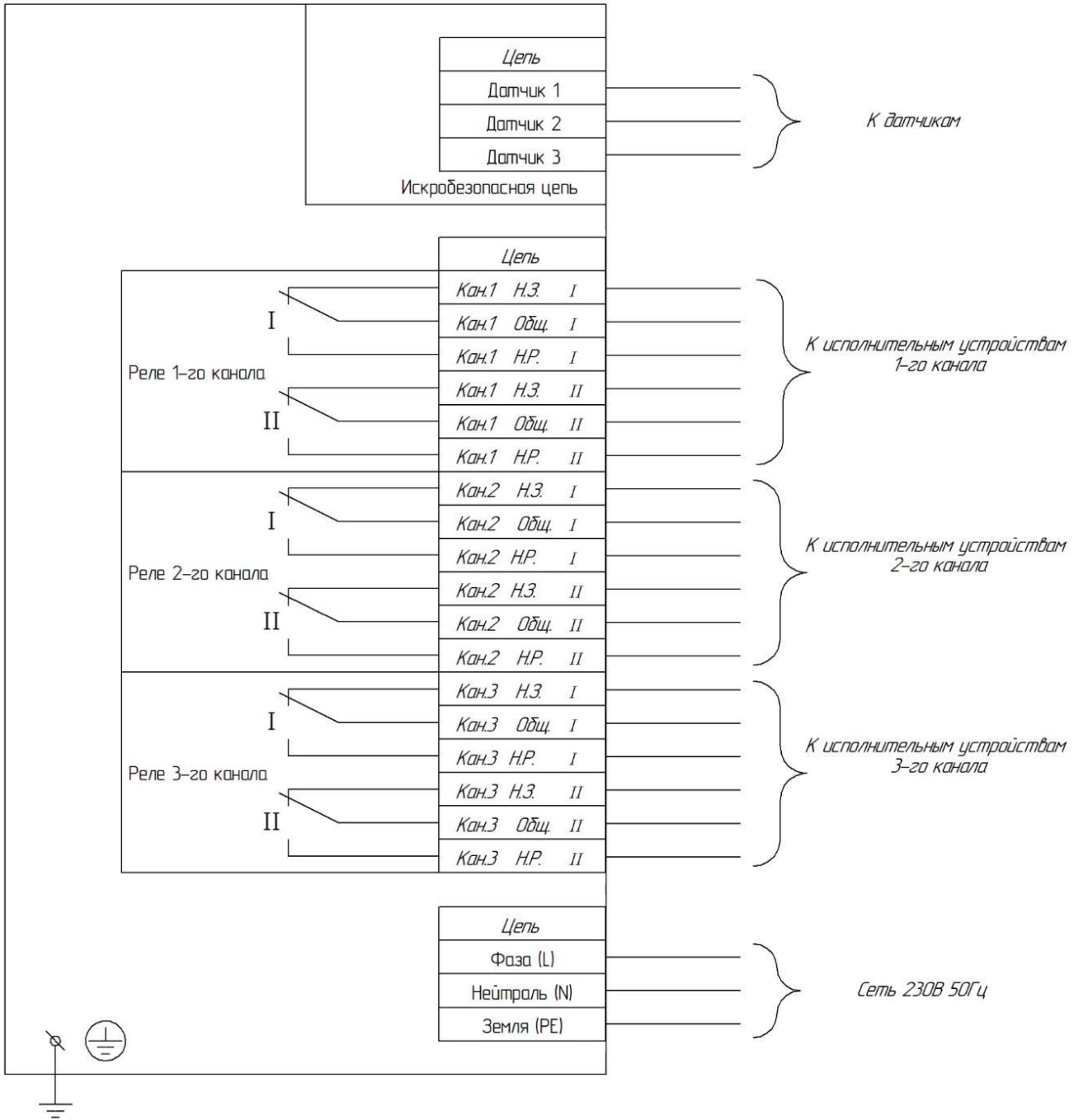
РИЗУР-300
