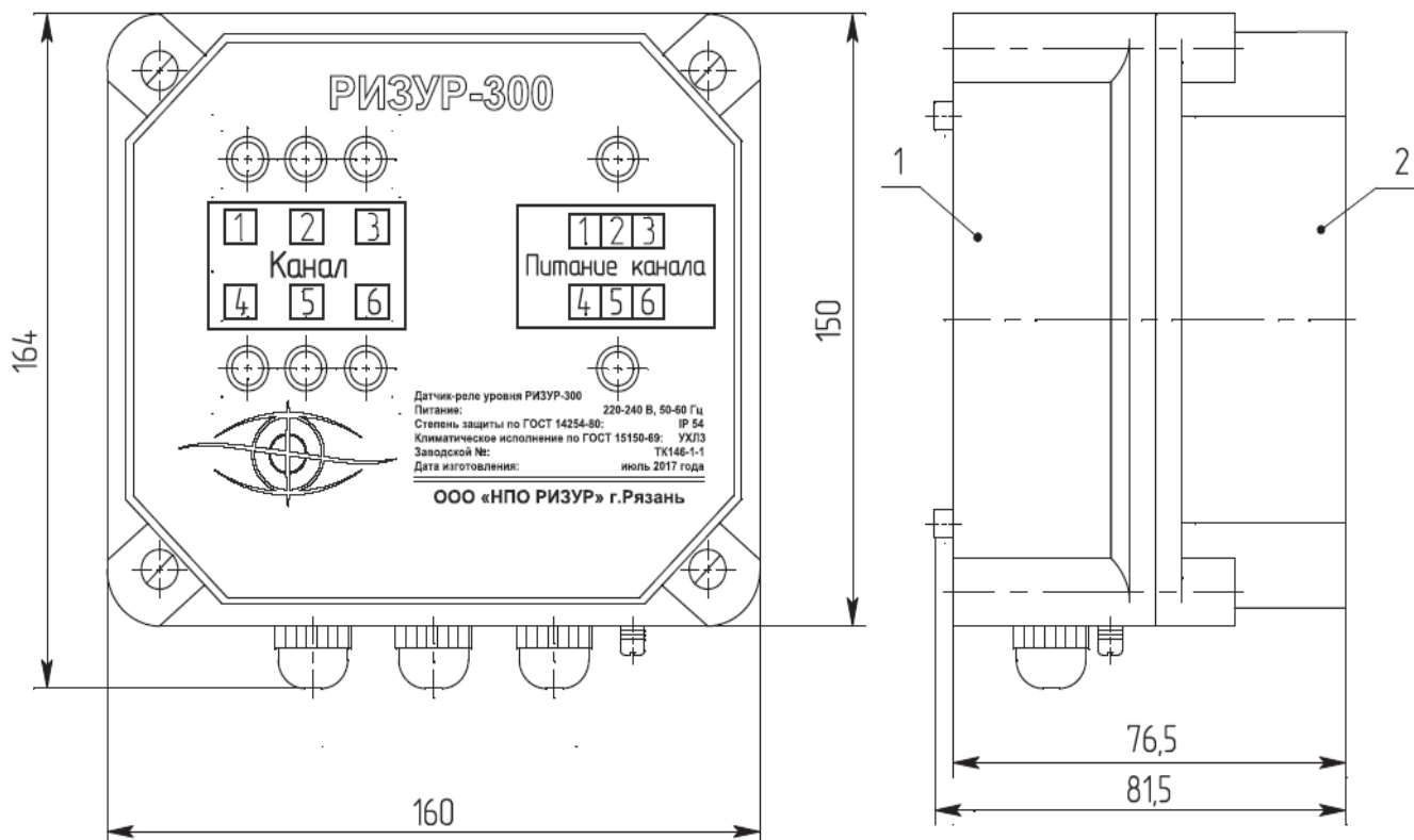
Рис.1.2. 4-6 датчика
