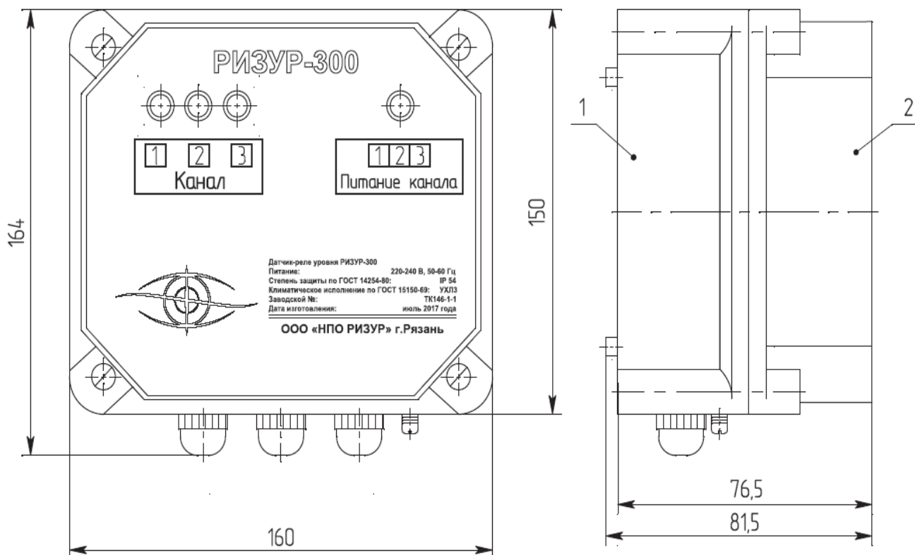
Рис.1.1. 1-3 датчика
