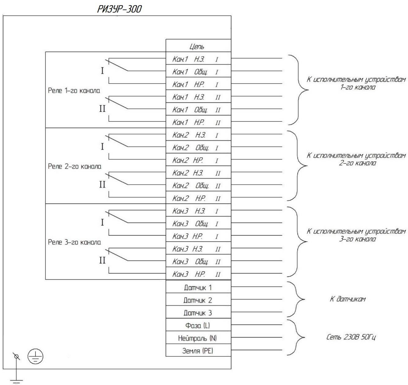
Рисунок 4.1 1-3 датчика
