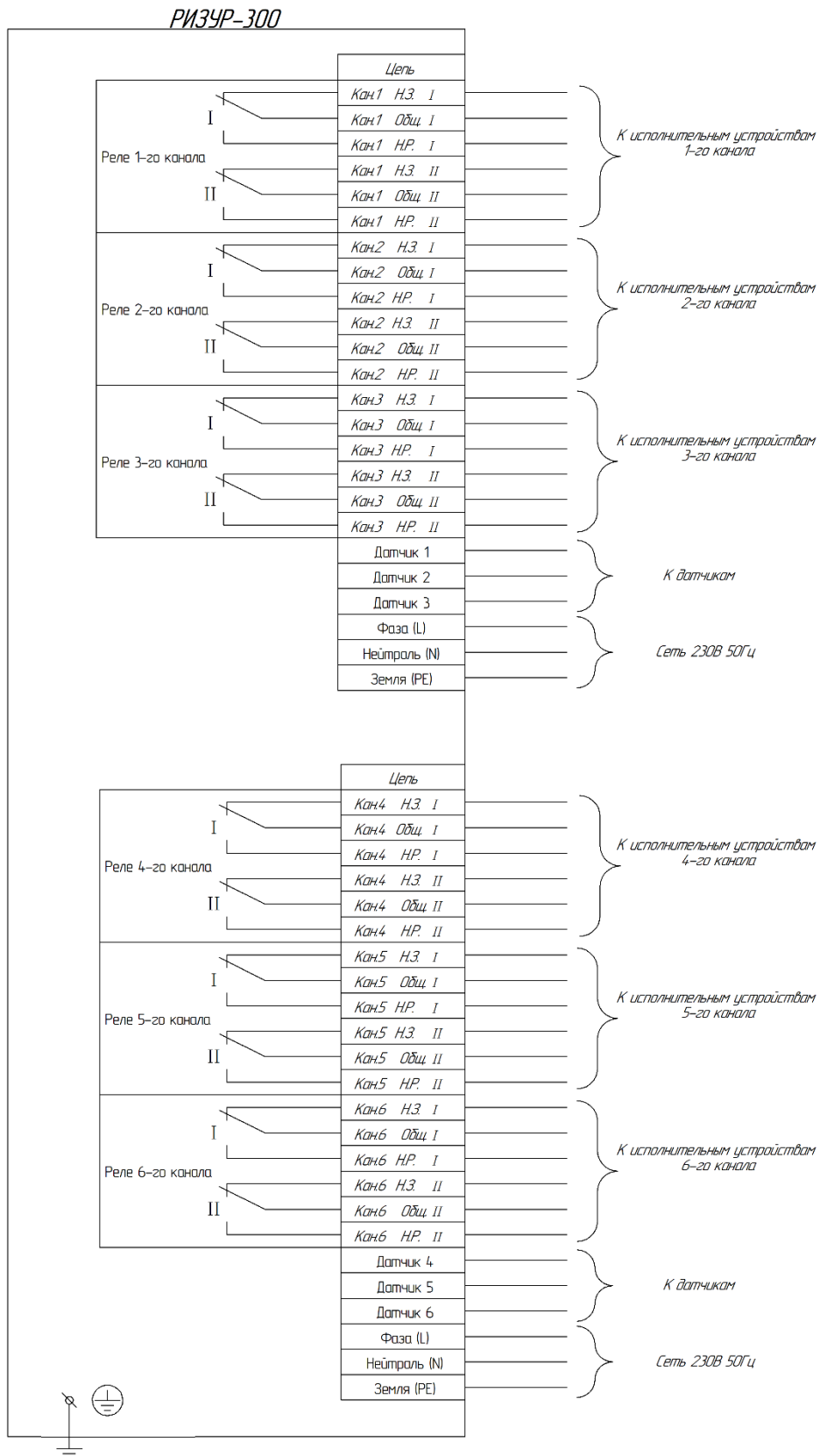
Рисунок 4.2 4-6 датчиков
