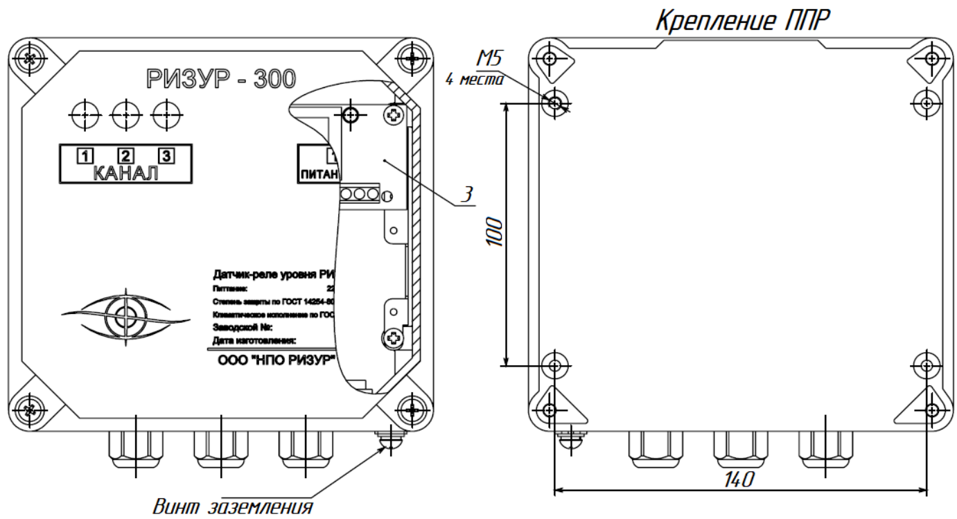
Рис.2.1. 1-3 датчика
