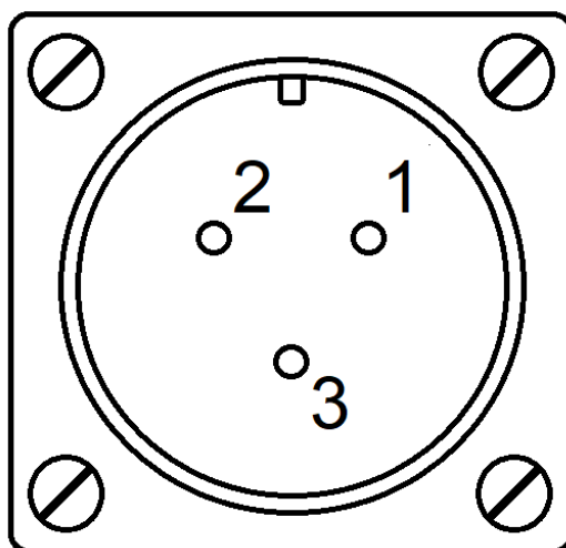
Рисунок В.1 Разъем подключения
