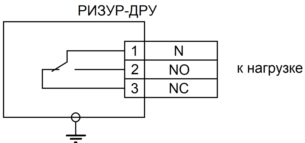
Рисунок В.2 Электрическая схема (исходное состояние – поплавок опущен)
