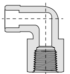
Фитинг угловой проходной под приварку внахлест с внутренней резьбой RizurLok-P-W-Pf
