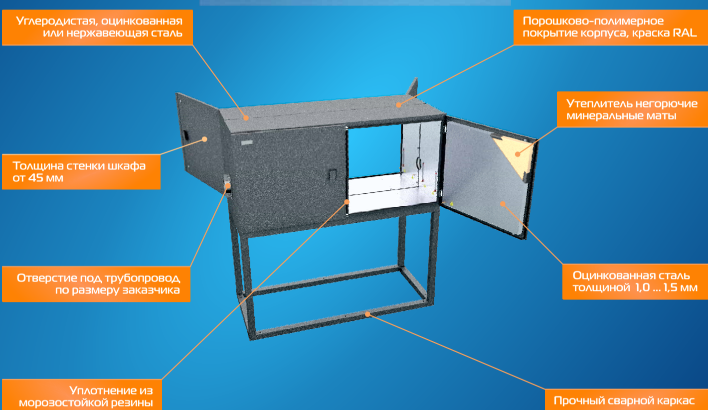
Термошкаф РизурБокс-М-РВ вертикально разъемный, 4х дверное исполнение
